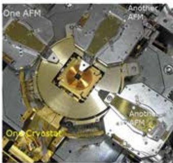
Multiprobe AFM
